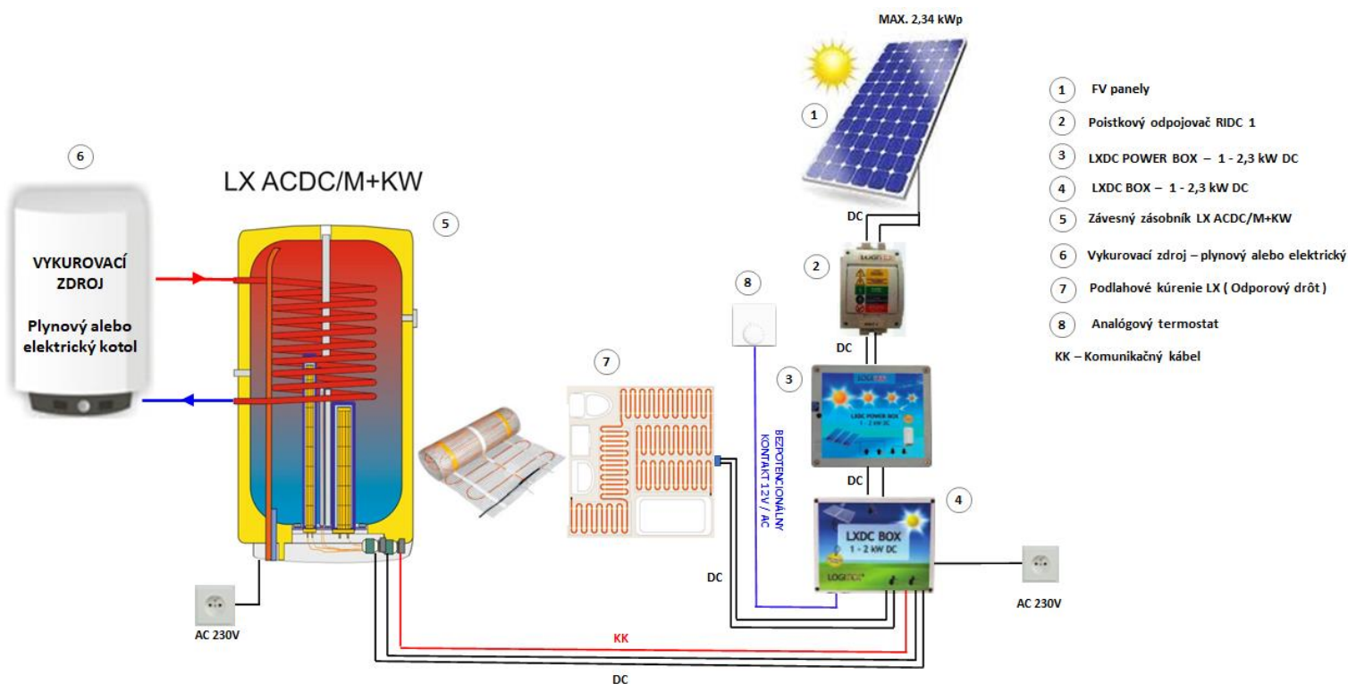
Ilustračné znázornenie zapojenia LXDC POWER BOX 1-2,3 kW DC.
